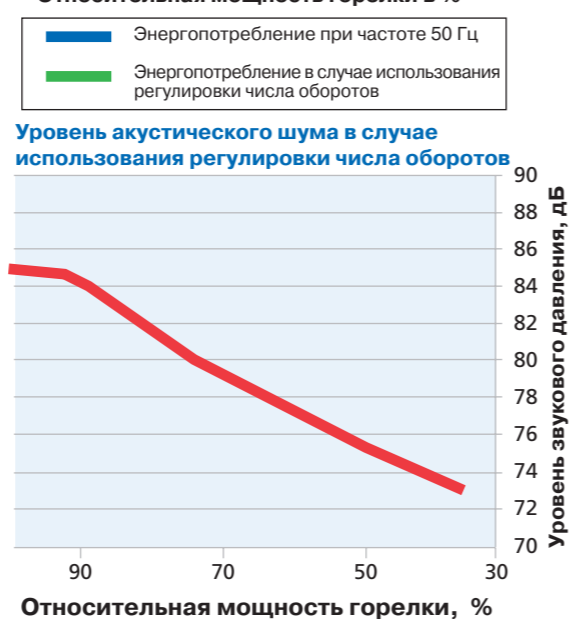
Уровень акустического шума в случае использования регулировки числа оборотов
